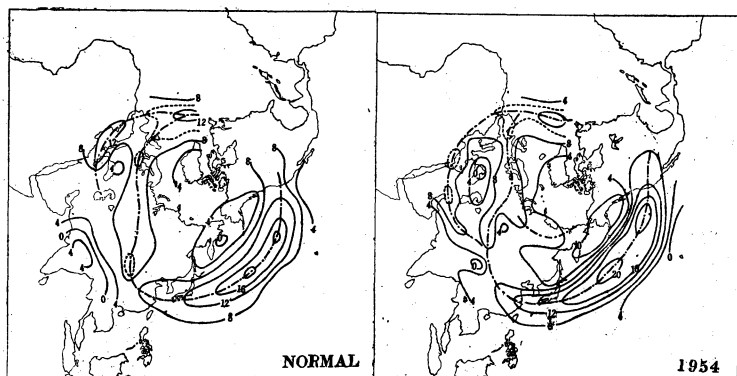
(a) (b) 第6図 500 mb 面における6月の偏西風の分布、(a) Normal, (b) 本年、実線は等風速線、鎖線は最強風速帯。(単位 m/sec)
