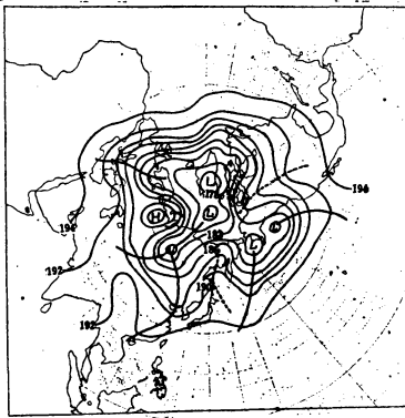
第7図 1953年7月15～19日の5日平均高度図。太線はトッブ・ライン、点線はリッジ・ライン。(単位は100フィート)
